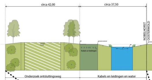
Profiel zuidzijde Nobelhorst - Oosterwold
